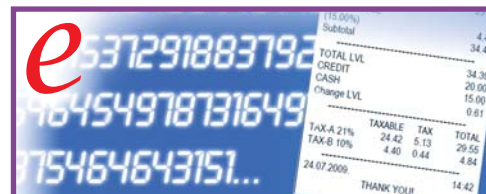
ELEKTRONISKAIS ŽURNĀLS
